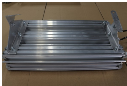
Кронштейн для крепления светильника к стене или к потолку
